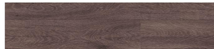
D3502 Dąb Olimpia | Olympia Oak | Дуб Олимпия
